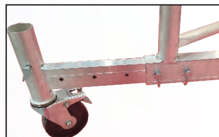
Разтегателна основа Retractable base
